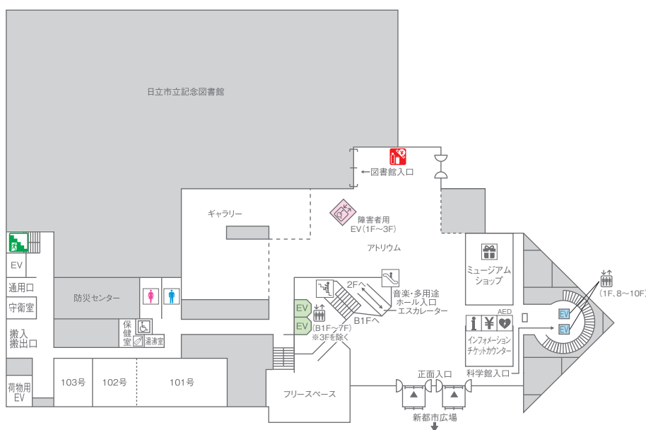
1F 平面図
